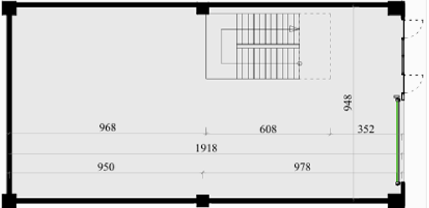
ZEMİN KAT
