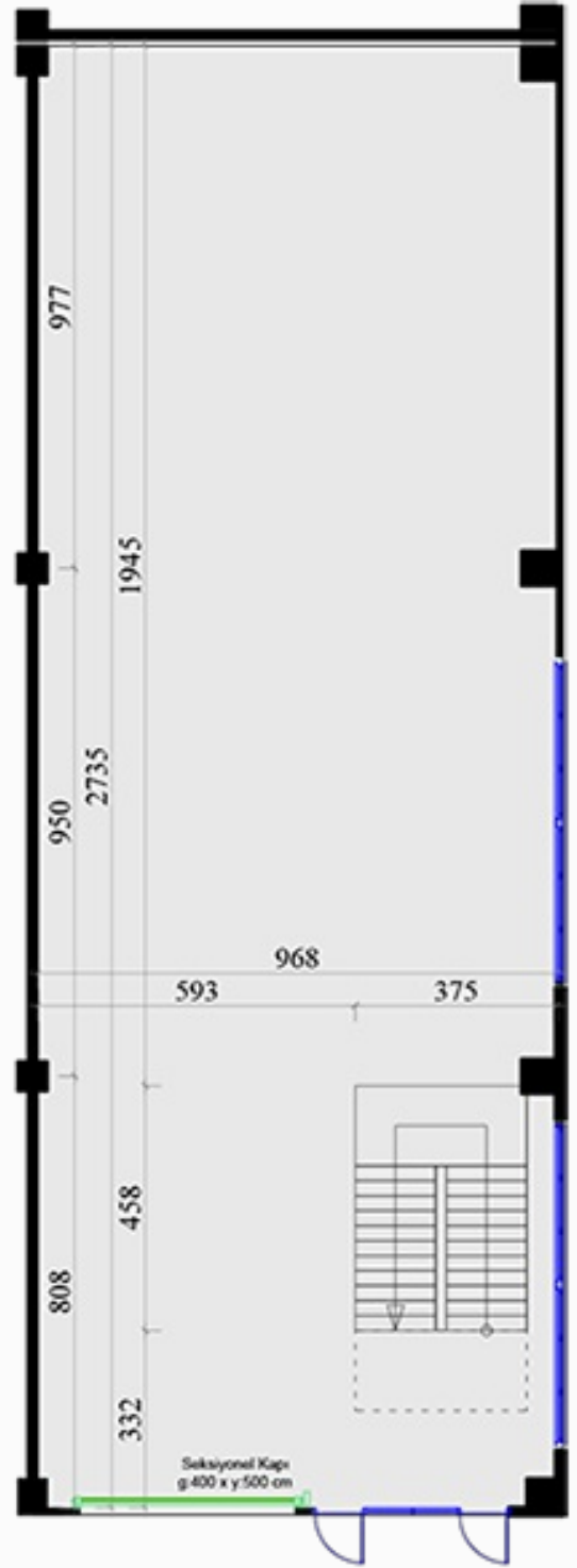
ZEMİN KAT
