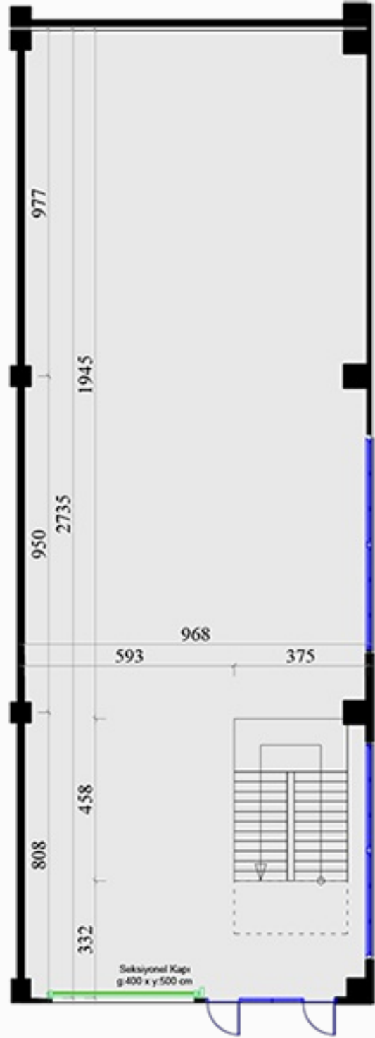
ZEMİN KAT
