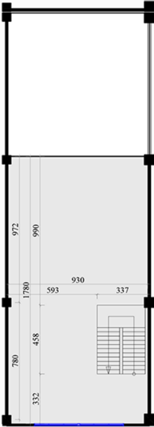
1.NORMAL KAT
