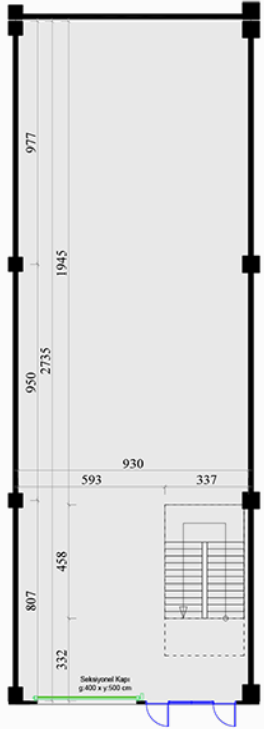
ZEMİN KAT
