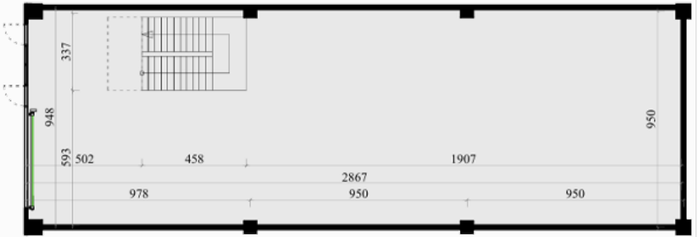
ZEMİN KAT
