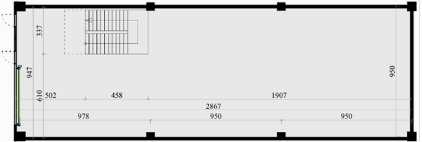
ZEMİN KAT
